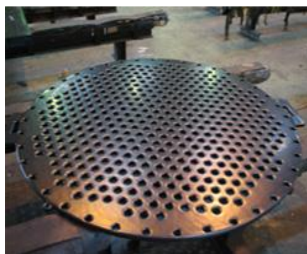
目皿ポリエチレンライニング
